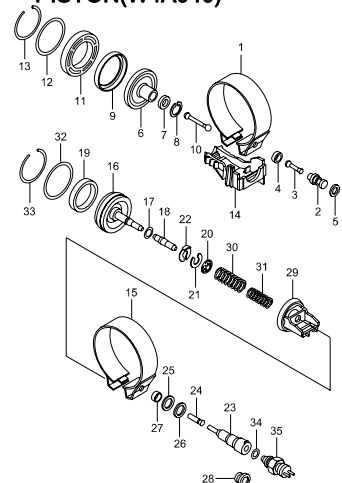
3615 BRAKE BAND & PISTON(W4A040)
