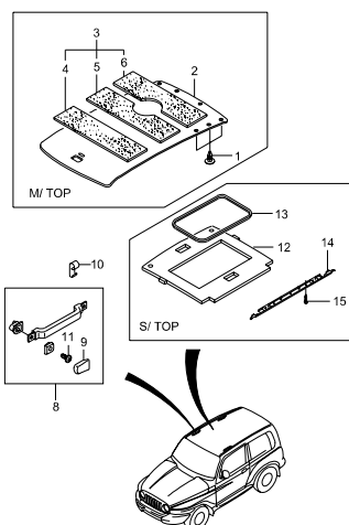
7330 HEADLINING
