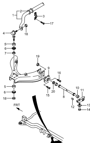
4420 STABILIZER BAR
