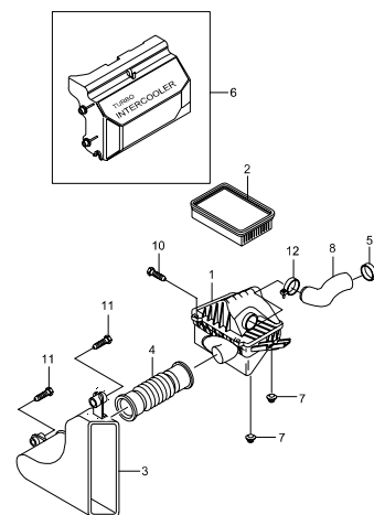
2311 AIR CLEANER(TURBO)
