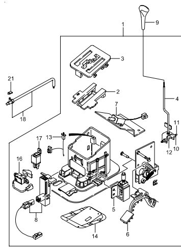
3731 AUTO SHIFT CONTROL(MB)
