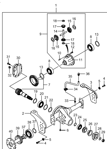
4120 FRONT AXLE(KSC)
