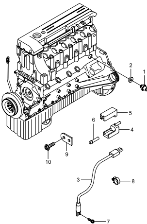
1420 SENDER UNIT & SWITCH(OM600)
