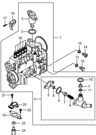
1810 INJECTION PUMP(OM600)
