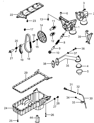
1531 OIL PAN & PUMP(E20,E23)
