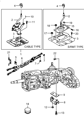
3710 MANUAL SHIFT CONTROL
