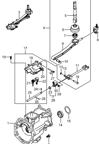
3154 SHIFTER & EXTENSION-T5(4WD)
