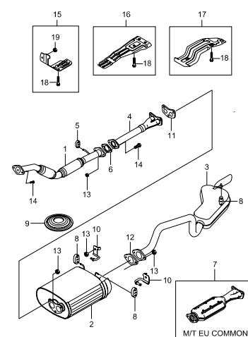
2411 EXHAUST SYSTEM(TURBO)
