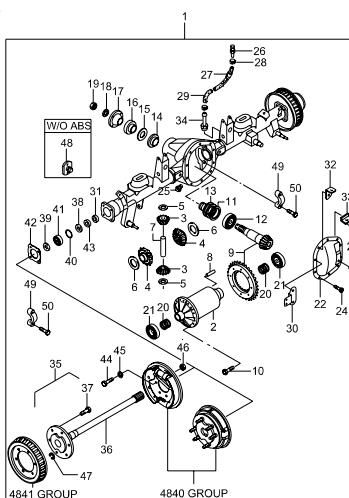
4210 REAR AXLE(KSC)
