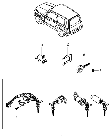
7010 KEY SET
