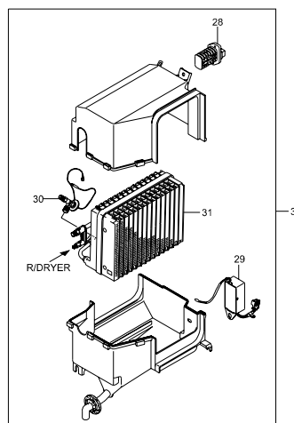
6840 EVAPORATOR
