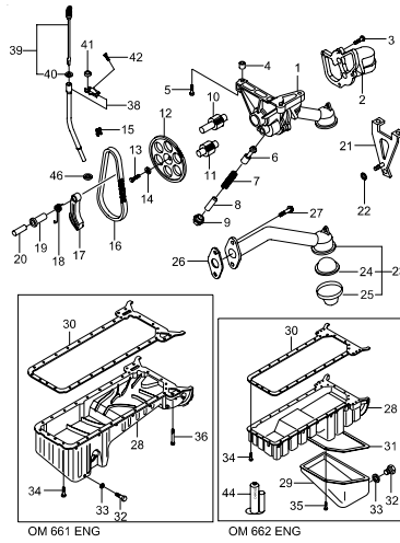
1530 OIL PAN & PUMP(OM600)
