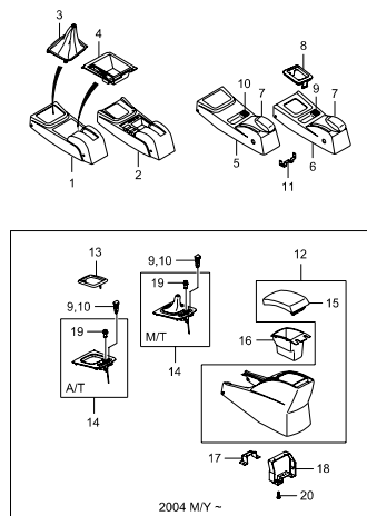
7630 CONSOLE
