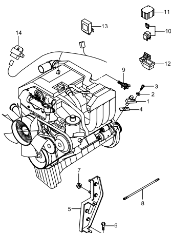
1430 SENSORS(GSL)
