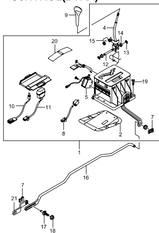
3740 AUTO SHIFT CONTROL(BTRA)
