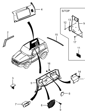
7730 PILLAR TRIM
