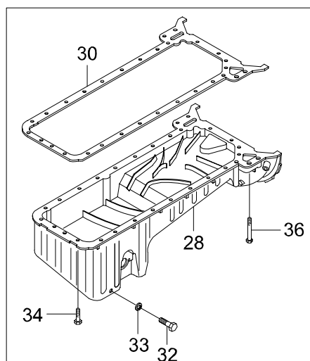
OM 661 ENG
