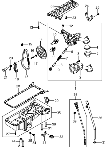
1532 OIL PAN & PUMP(E32)
