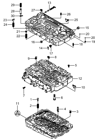
3613 VALVE BODY(W4A040)
