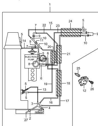
1621 VACUUM SYSTEM(OM600;MB A/T)
