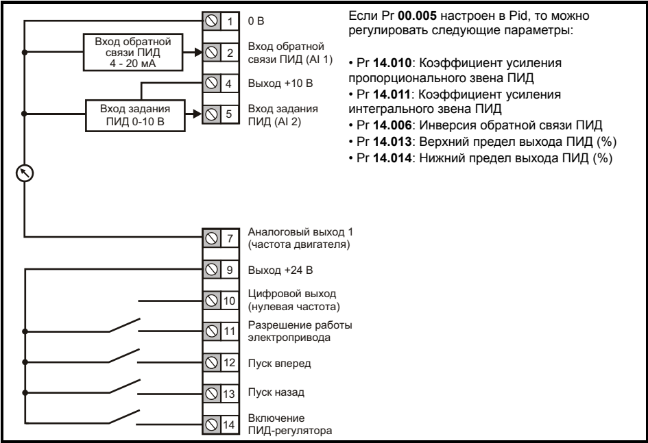
Рис. 4-18 Pr 00.005 = Pid (60 Гц)
