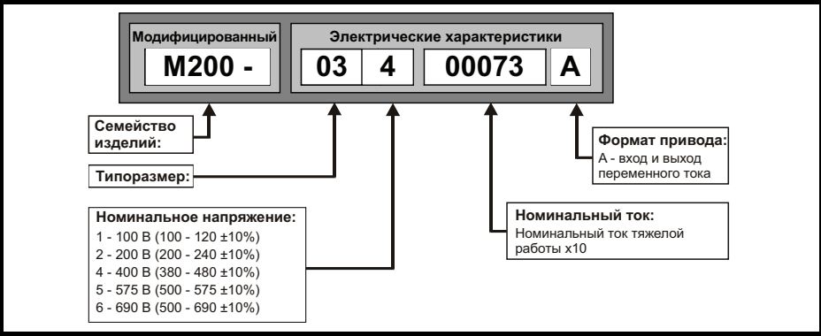
Рис. 1-1 Структура номера модели
