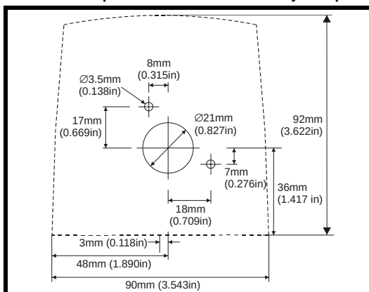
Figure 4-1 Panel cut-out / Découpe du panneau / Aussparung für Montage an der Schaltschranktür / Apertura sagomate per il montaggio a pannello / Hueco de montaje del panel
