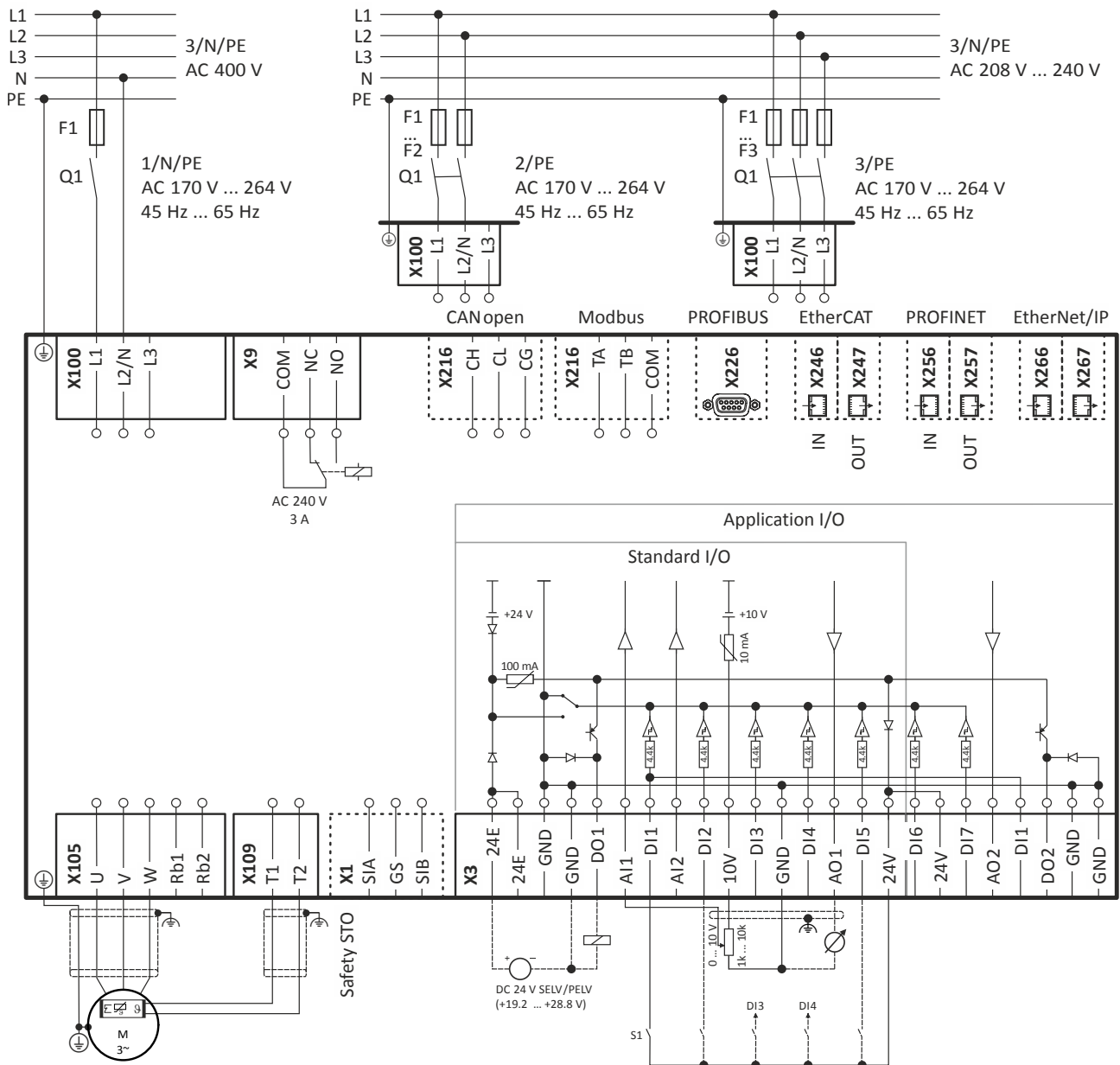
Fig. 4: Wiring example
